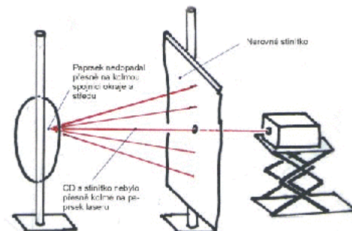
Obrázek 3: Experimentální sestava
