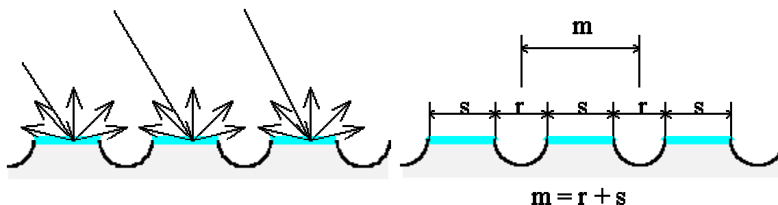
Obrázek 1: CD jako difrakční mřížka
