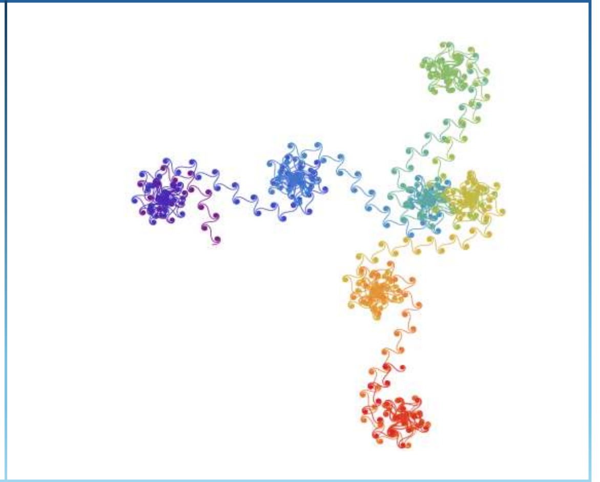
Obrázek 2: Spirála s parametrem \phi
