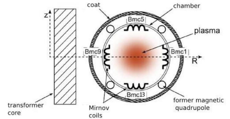
Obr. 5 Mirnovovy cívk
